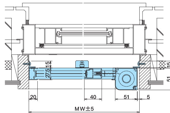
横断面 (片引き)
