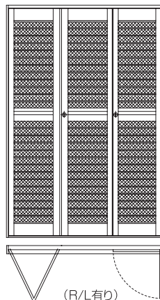
VFタイプ (折戸+小扉)
